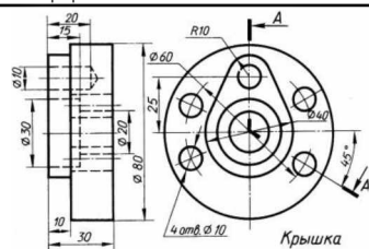
Деталь «крышка»
