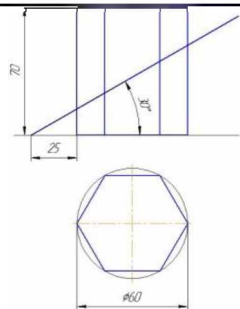
Пересечение призмы проецирующей плоскостью
