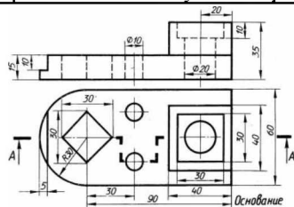
Деталь «основание»
