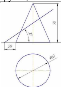
Пересечение конуса проецирующей плоскостью
