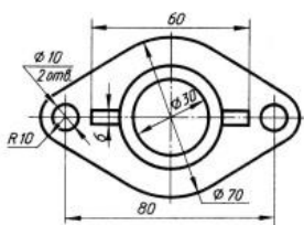
Деталь «крышка»
