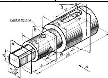
Деталь «вал»
