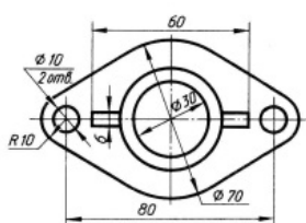
Деталь «крышка»
